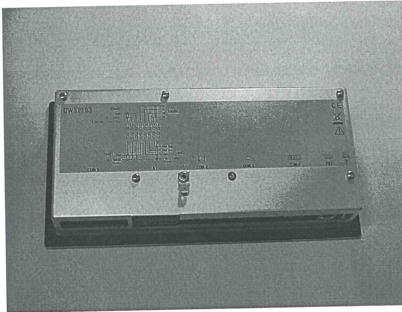
Abbildung / figure 2: Rückseite / rear side DWS2103
